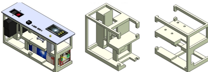
FIGURA 8. Diseño 3D de estructura interna para anclaje de equipos con maleta
