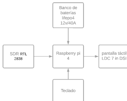
FIGURA 7. Diagrama de bloques del diseño del prototipo
