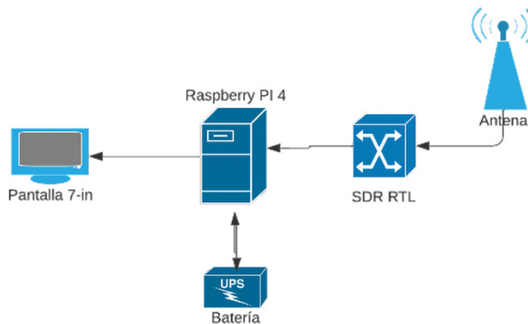
FIGURA 3. Diagrama de Módulos con referencia de equipos
